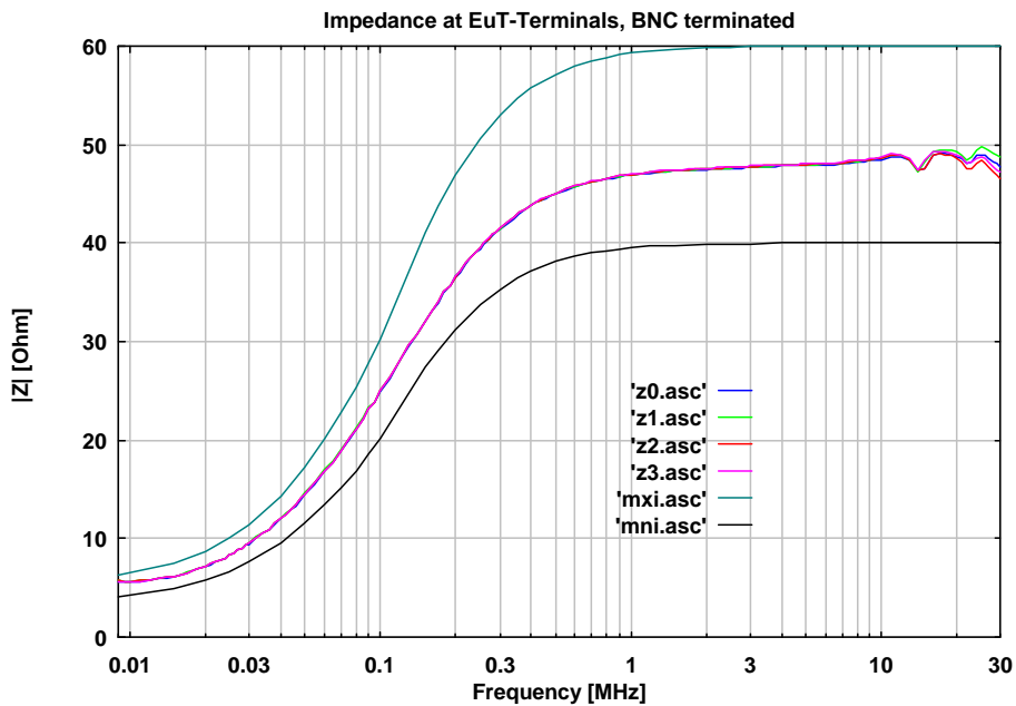
Abb. 4 Impedanz an den Prüflingsklemmen (CEKON), BNC mit 50 Ω Abschluss Impedance of connector for DuT (CEKON), BNC terminated with 50 Ω
